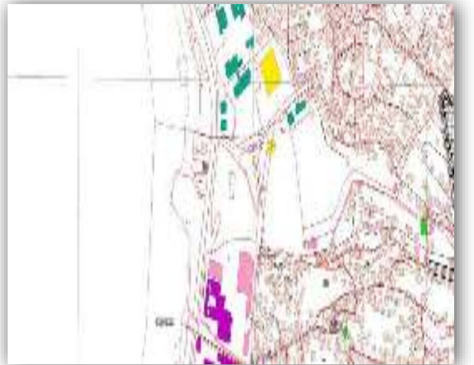
Sultaniye Çayırı içerisinde bulunan namazgaha ait rölöve, restitüsyon ve restorasyon projesi
